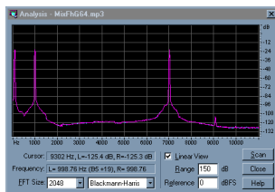
FHG 64kb/s (! andere Skala !)
