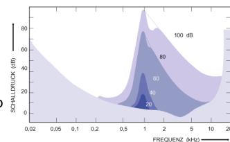
Die Maskierung eines 1 kHz Tons mit der angegebenen Lautstärke
