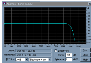
Frequenzverlauf bei 22,05kHz Samplingrate
